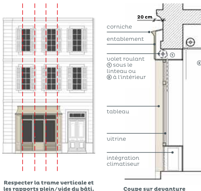
Coupe sur devanture
